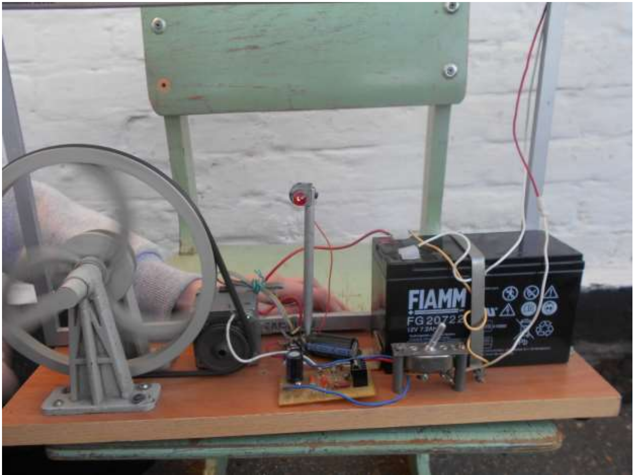
Преобразование механической энергии в электрическую
